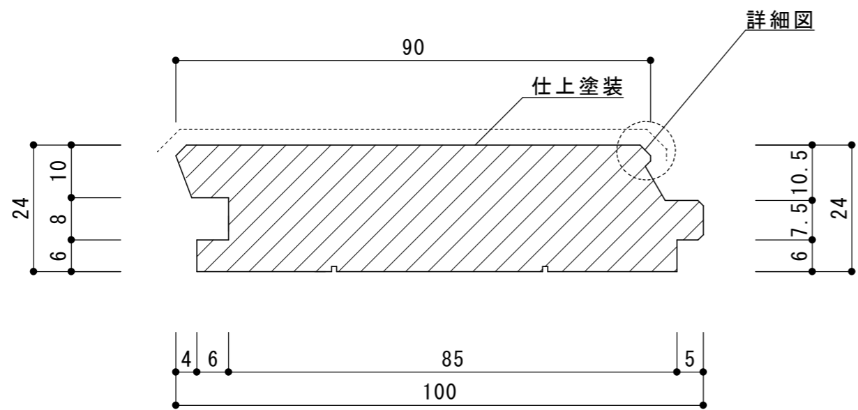
姿図
